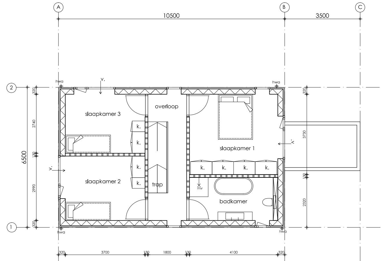
1e verdieping
