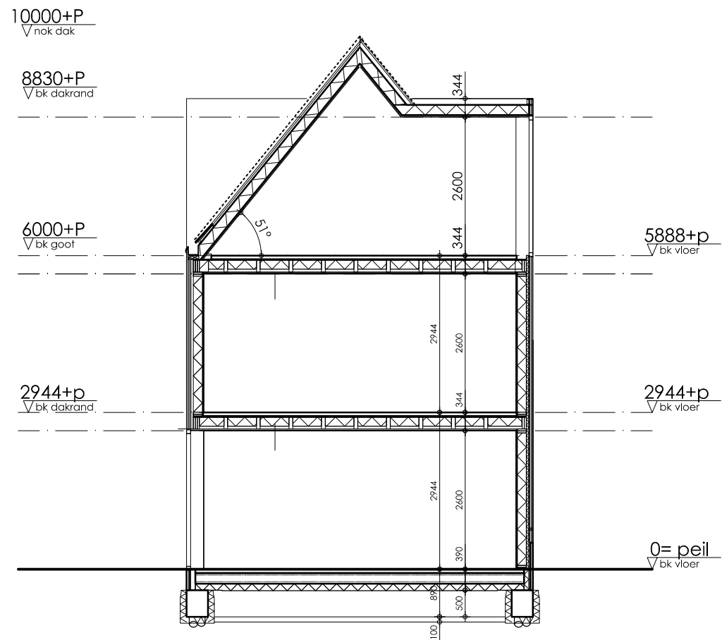
doorsnede woning
