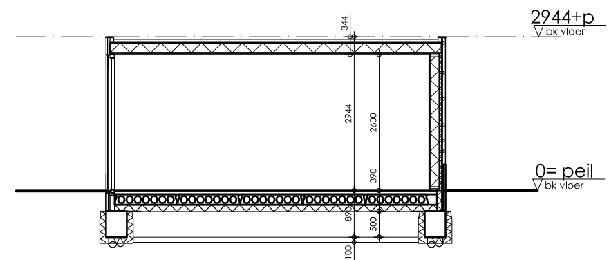
doorsnede garage
