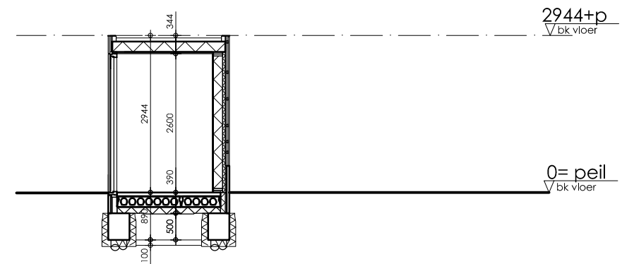
doorsnede berging
