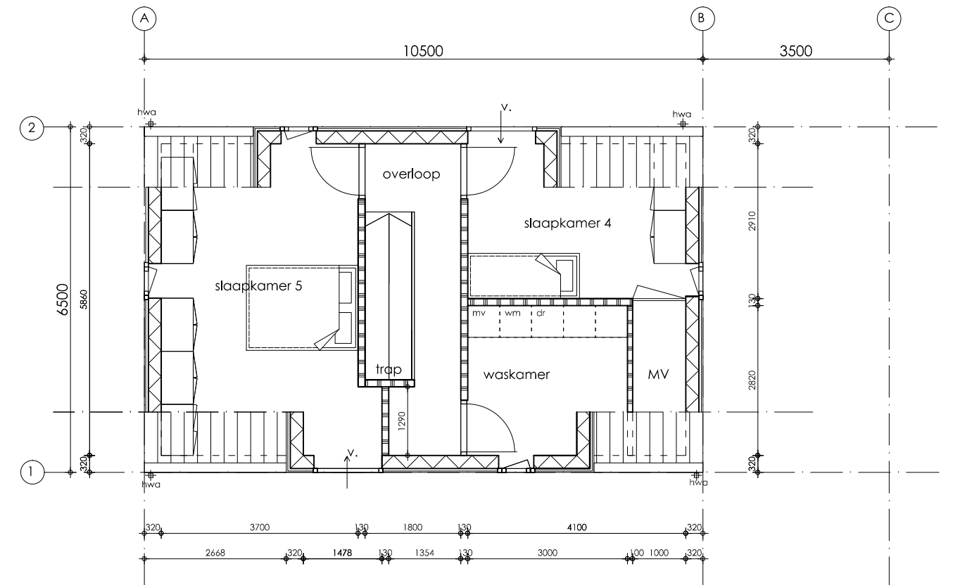
2e verdieping
