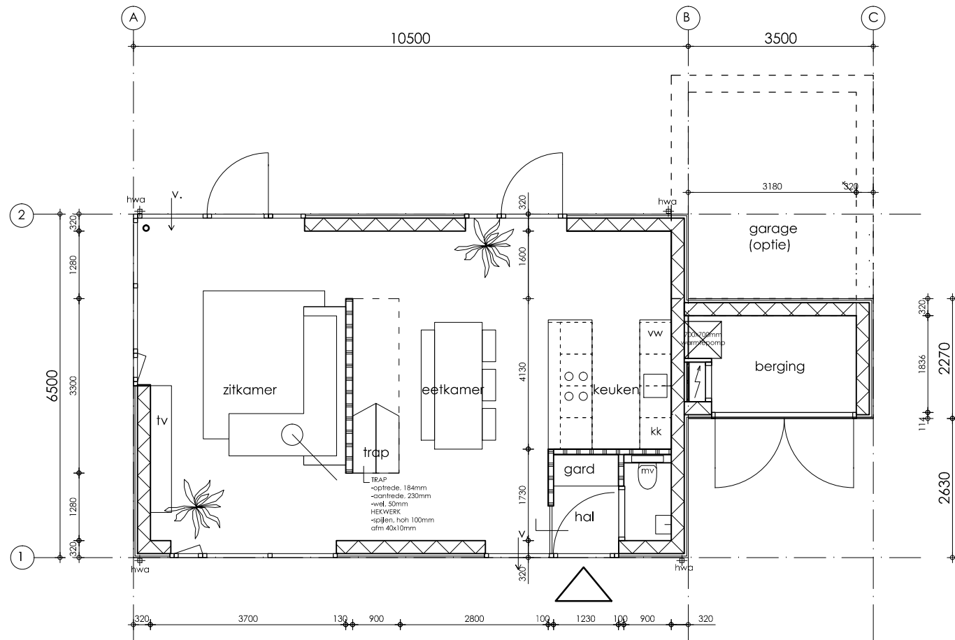
begane grond
