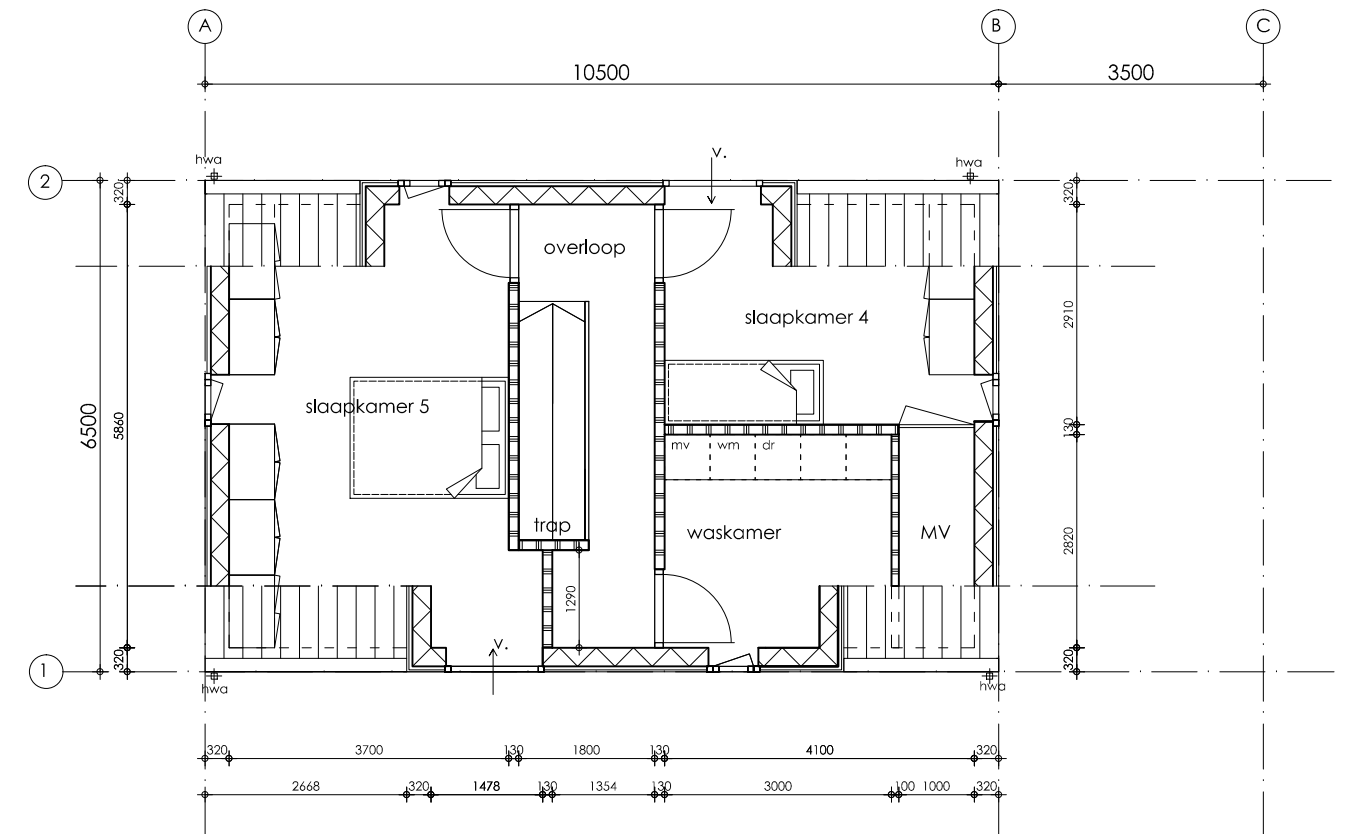
2e verdieping
