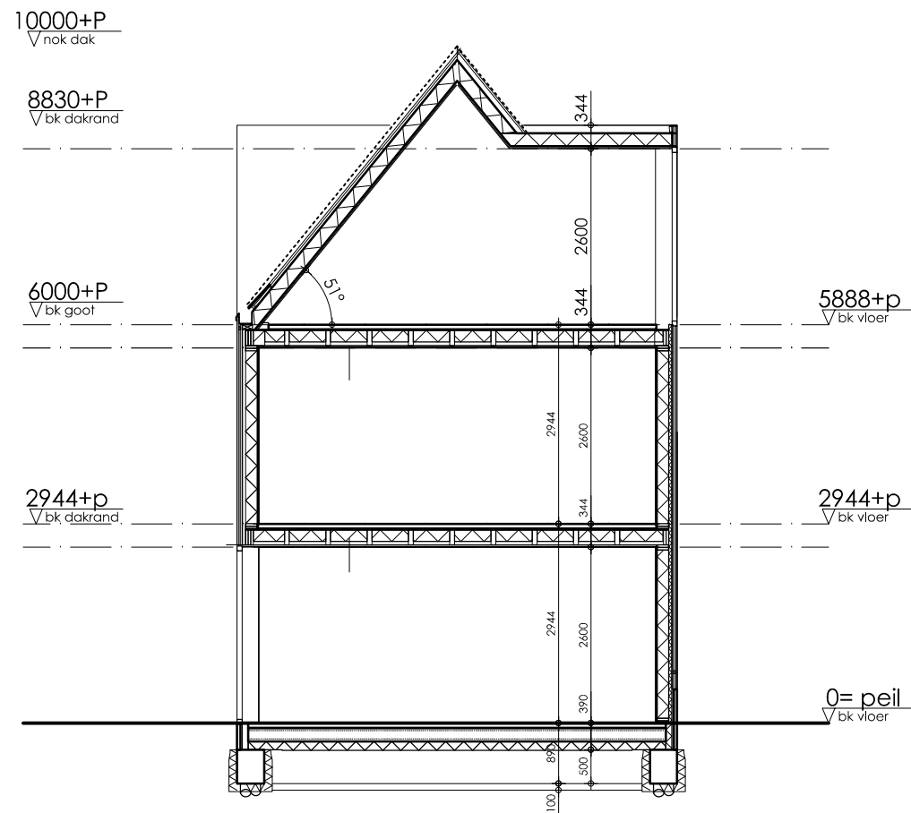
doorsnede woning
