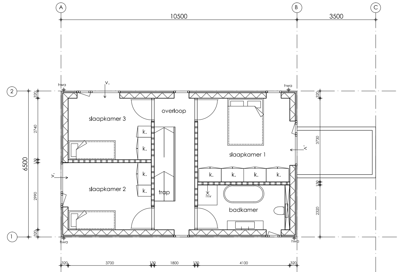
1e verdieping
